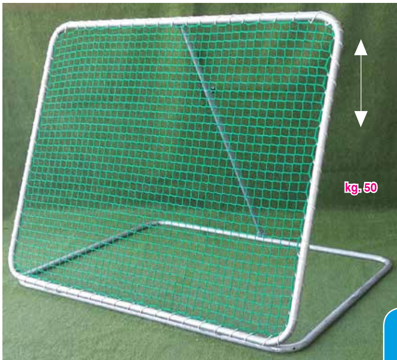
Art. 5041 Telaio con rete cm. 315 x 230 in ferro zincato ad inclinazione regolabile, per allenamento portieri e giocatori Iron frame with net, in galvanized iron dimensions 315 x 230 cm. adjustable inclination for goalkeepers and players
